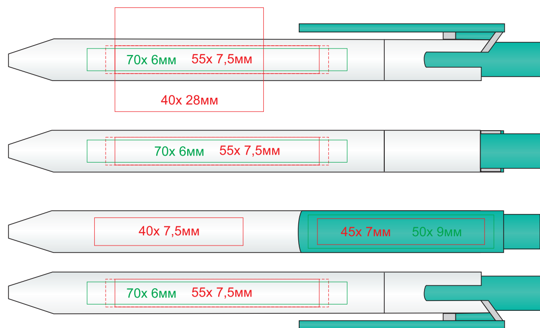
192/01/18 круговая шелкография
