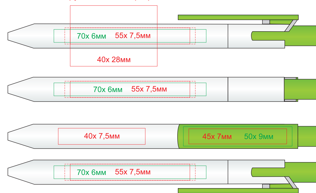
192/01/142 круговая шелкография
