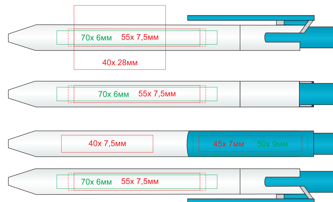
192/01/135 круговая шелкография
