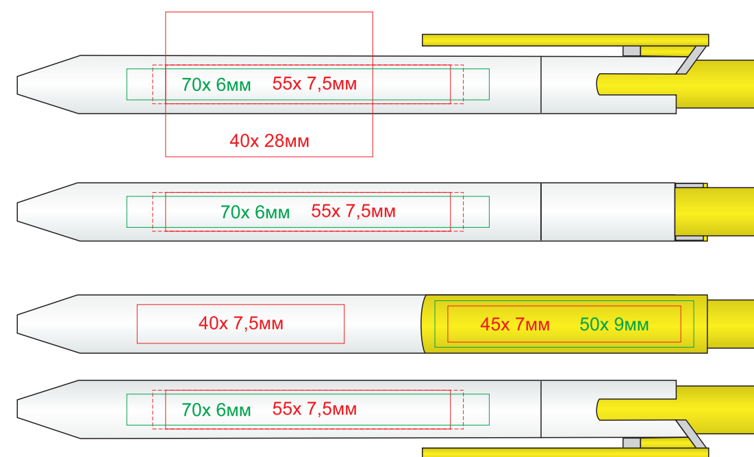
192/01/120 круговая шелкография
