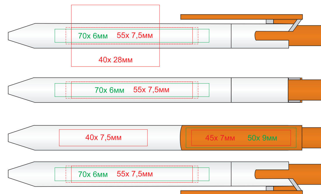
192/01/05 круговая шелкография
