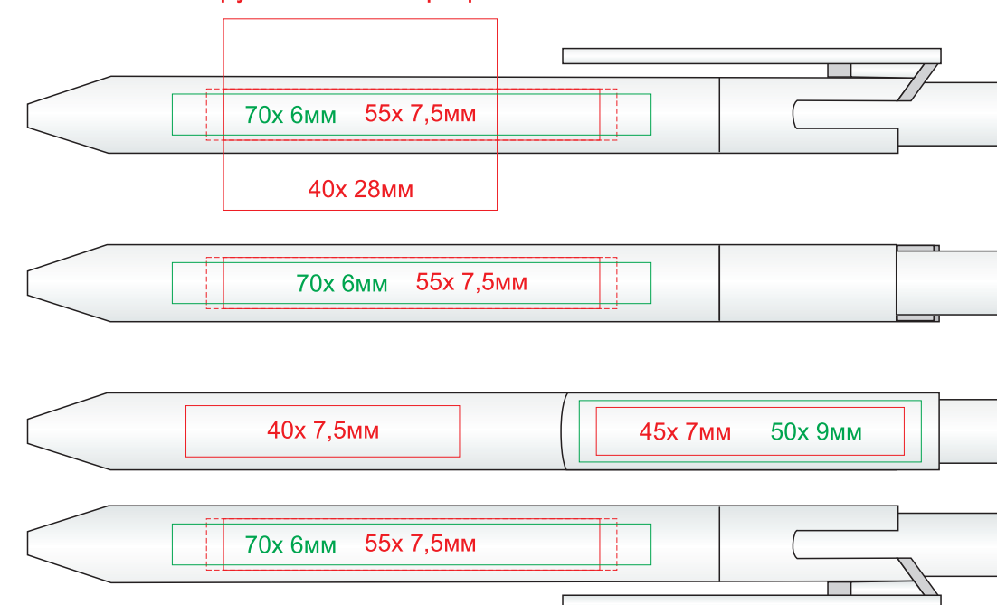
192/01/01 круговая шелкография
