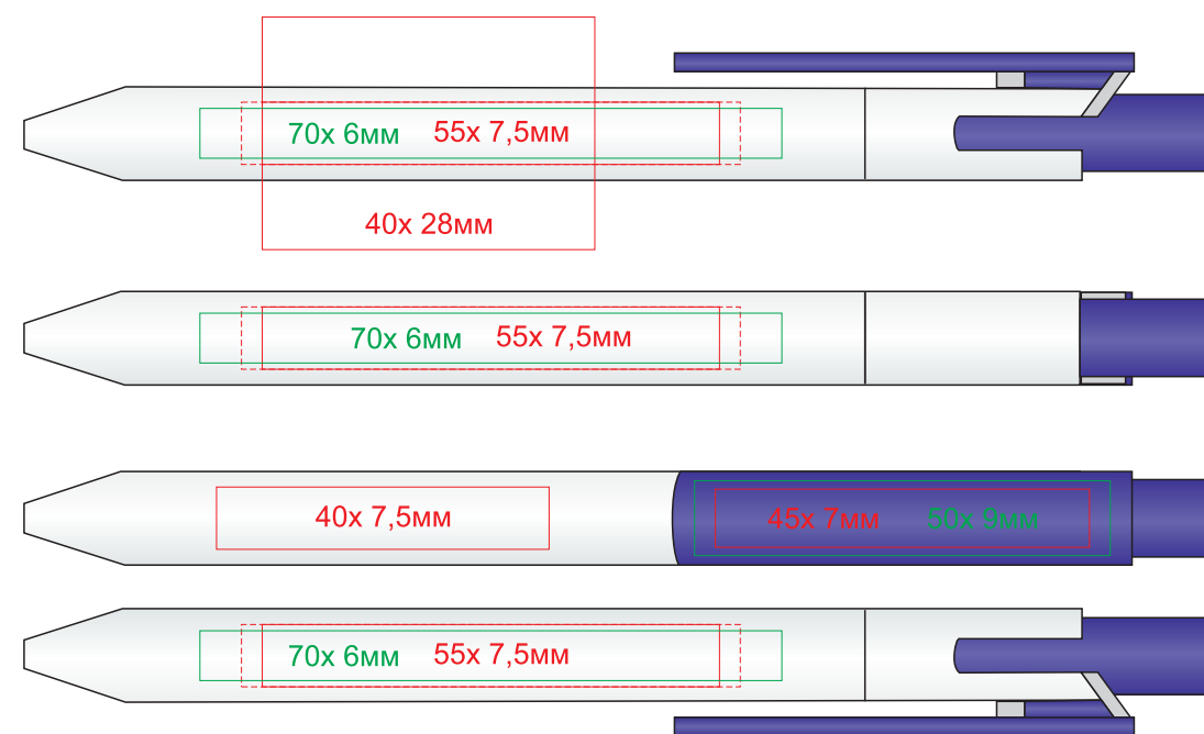
192/01/135 круговая шелкография
